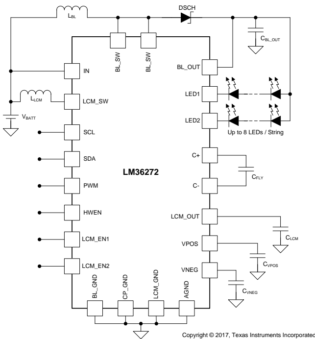
概略回路図
