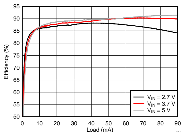
バックライト効率、3P7S
