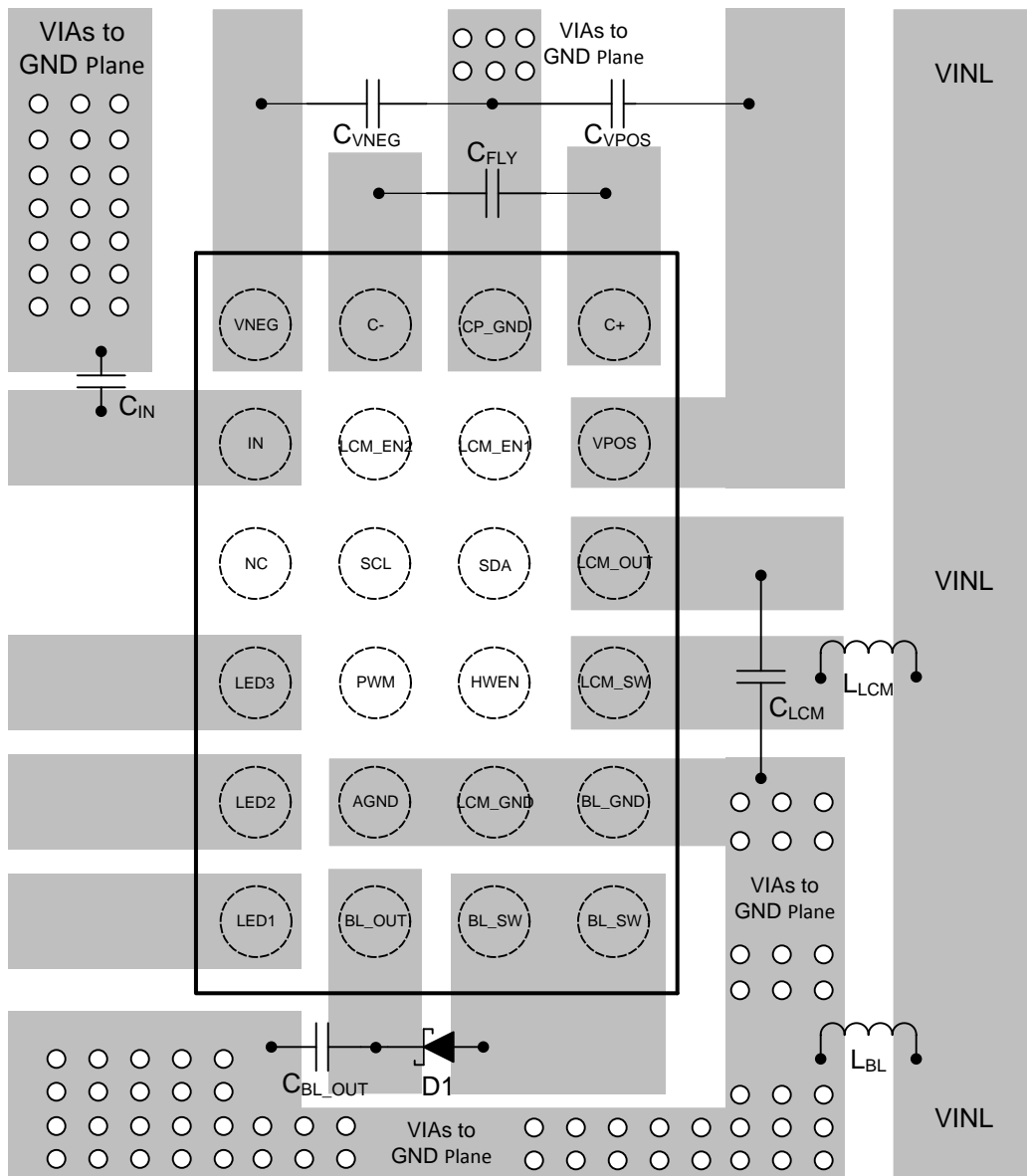
FIG 175. LM36273 Layout Example
