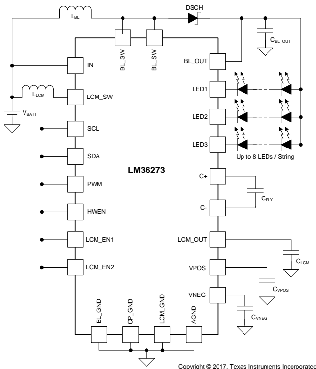
概略回路図
