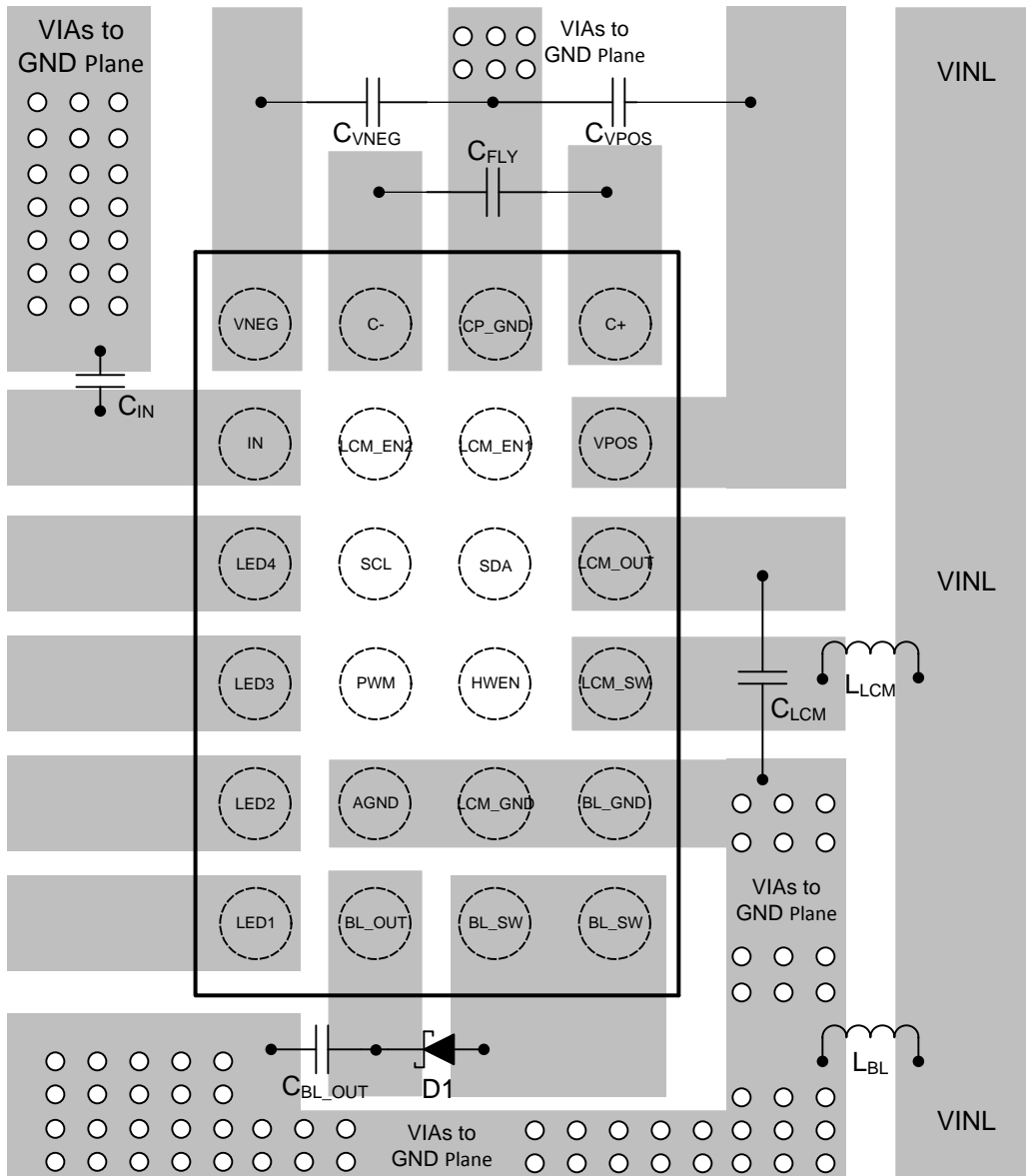
☒ 211. LM36274 Layout Example
