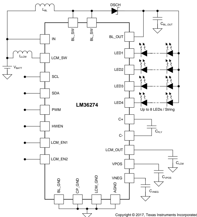
概略回路図
