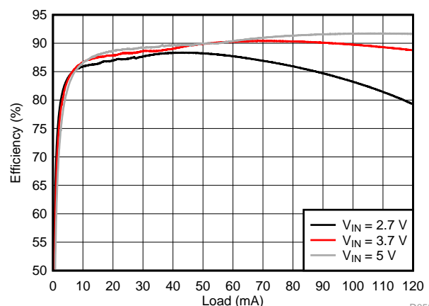
バックライト効率、4P6S
