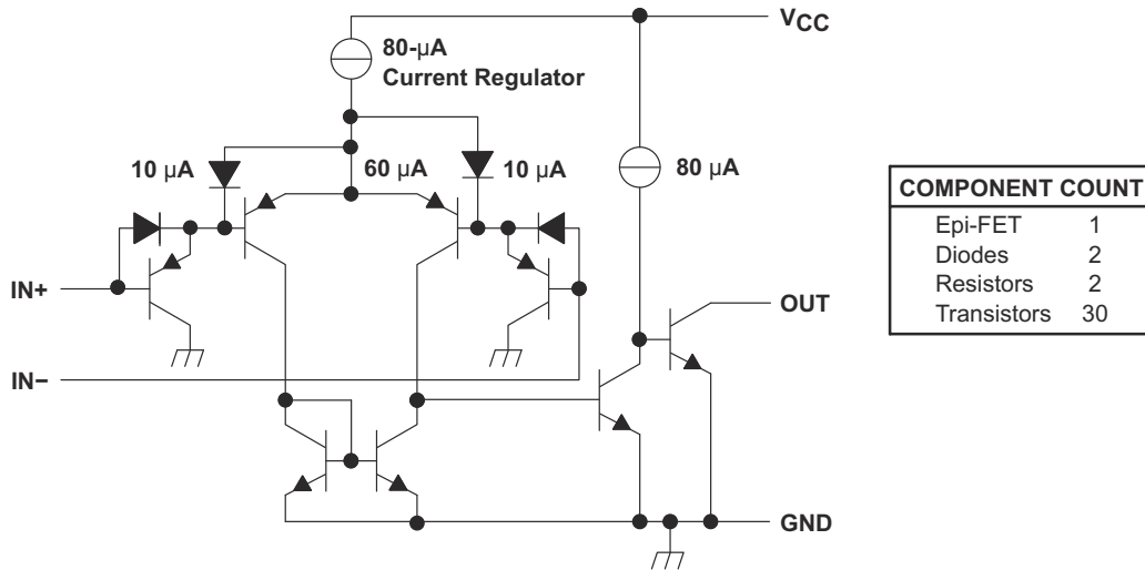
図 7-1. 回路図 (各コンパレータ)
