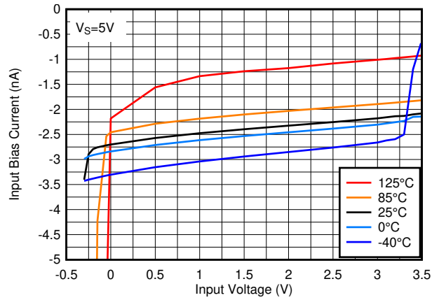
図 6-21. 入力バイアス電流と入力電圧との関係、5V
