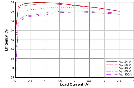
代表的な応用回路の効率、V OUT = 12V
