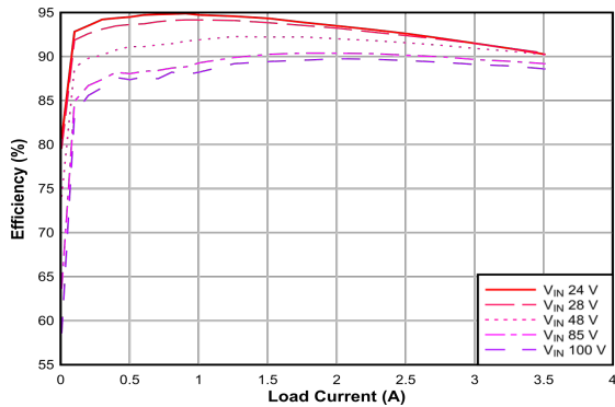
6-1. Conversion Efficiency (Linear Scale)
