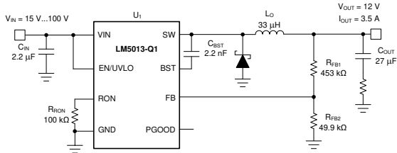
代表的なアプリケーション
