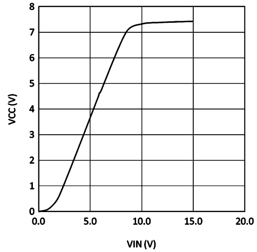
6-2. V_{CC} vs V_{IN}
