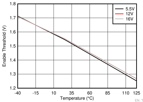
6-10. Enable Threshold
