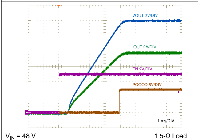
图 9-21. ENABLE ON, 10-A Resistive Load
