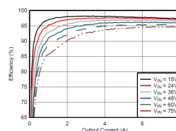
代表的なアプリケーション回路と効率特性、 V_{OUT} = 12V 、 F_{SW} = 400kHz
