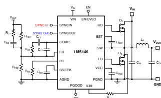
代表的なアプリケーション回路と効率特性、 V_{OUT} = 12V 、 F_{SW} = 400kHz
