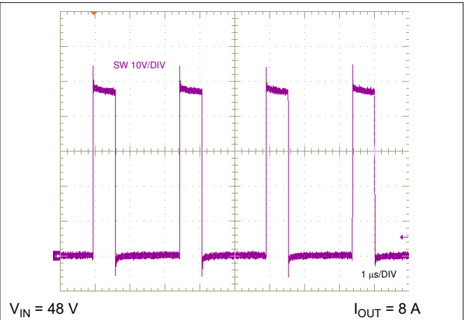
图 9-18. SW Node Voltages
