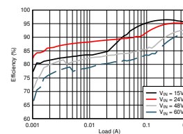
代表的な応用回路の効率、V OUT = 12V
