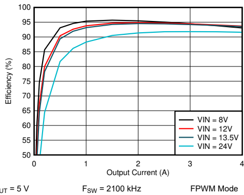
图 9-7. LM61440-Q1 Efficiency
