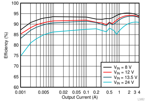
图 9-6. LM61440 Efficiency
