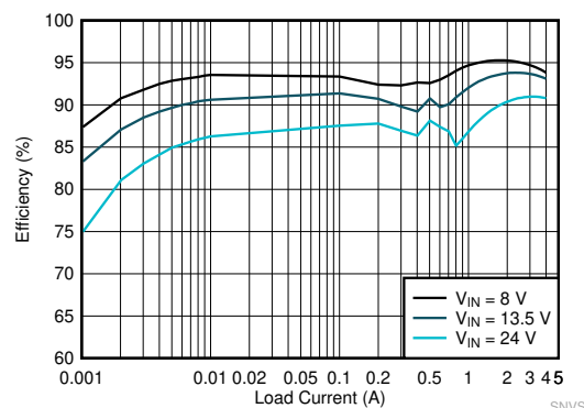
効率 : V_{\text{OUT}} = 5\text{V} 、 f_{\text{SW}} = 2200\text{kHz}
