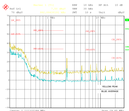
伝導 EMI : V_{\text{OUT}} = 5\text{V} 、 f_{\text{SW}} = 2100\text{kHz}
