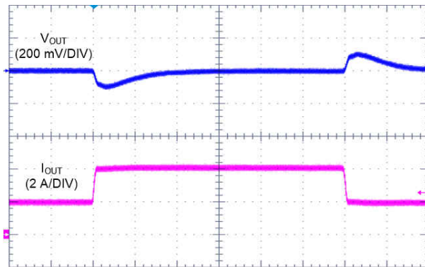
FIG 10-31. LM61440-Q1 Load Transient
