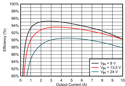
EVM の効率: V_{OUT} = 5\text{V} , F_{SW} = 2.2\text{MHz}
