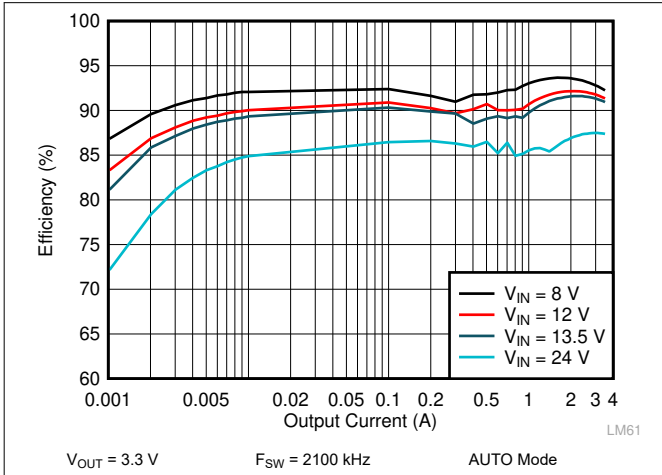
图 9-5. LM62435-Q1 Efficiency
