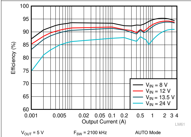
图 9-7. LM62435-Q1 Efficiency
