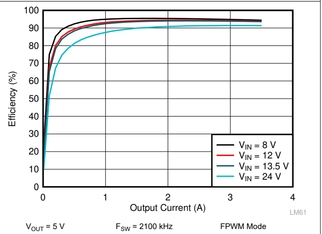
图 9-8. LM62435-Q1 Efficiency
