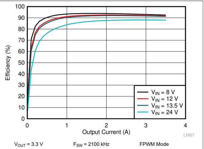
图 9-6. LM62435-Q1 Efficiency
