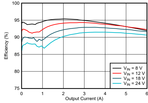
効率プロット、V OUT = 5V、f SW = 2.1MHz
