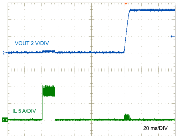
図 9-9. LM63460-Q1 Short-Circuit Recovery to No Load
