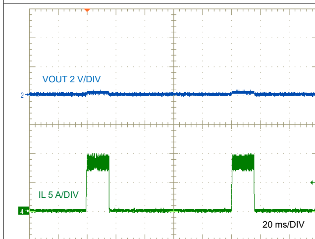
図 9-27. LM63460-Q1 Short Circuit Hiccup
