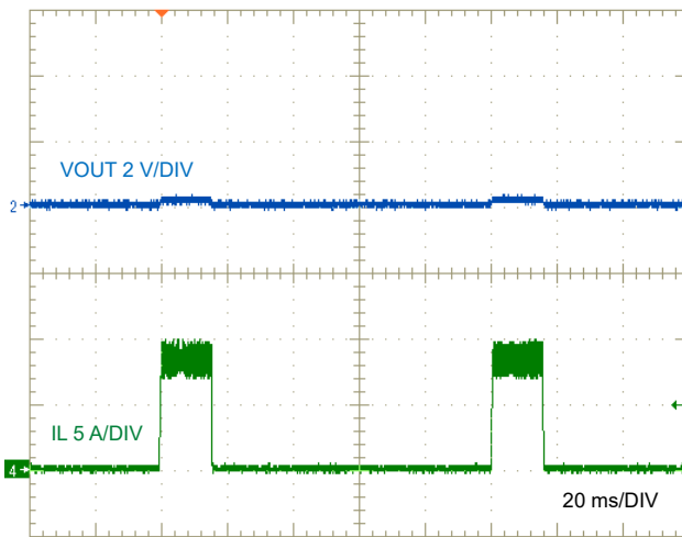
8-28. LM634x0-Q1 Short-Circuit Hiccup
