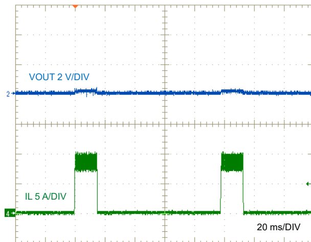
図 9-8. LM63460-Q1 Short-Circuit Hiccup
