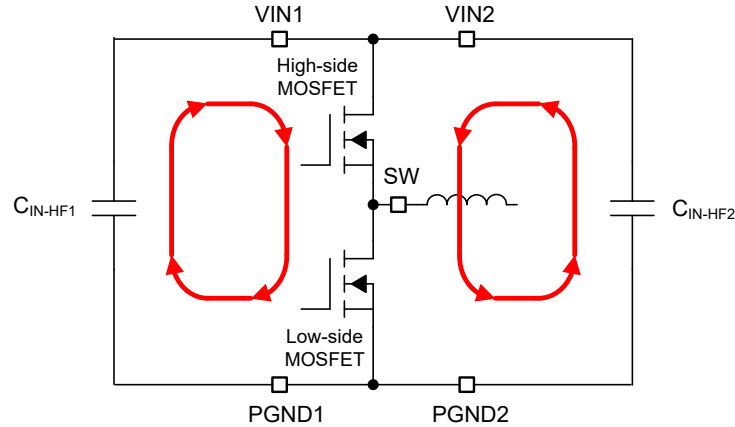
図 8-30. Input Current Loops
