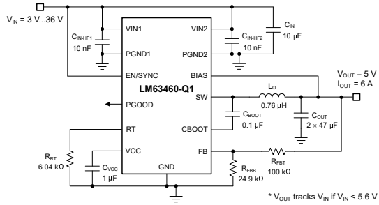
代表的な回路図
