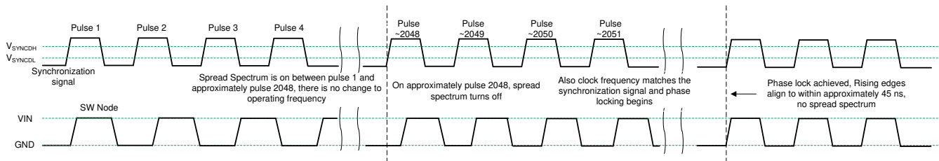
図 8-3. Synchronization Process
