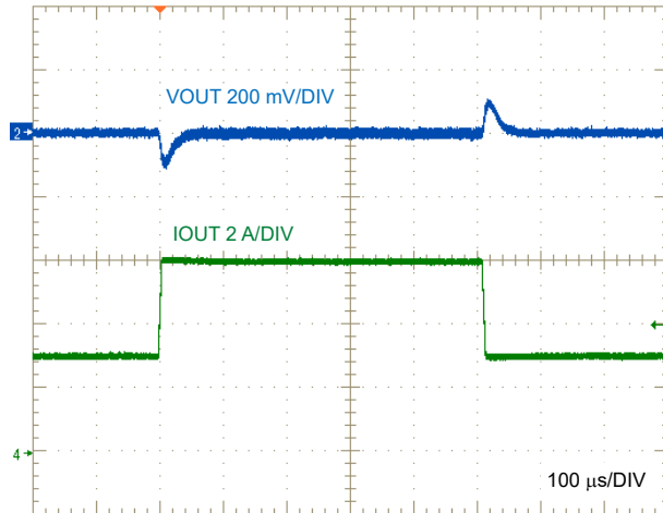
図 9-6. LM63460-Q1 Load Transient, I_{OUT} = 3\text{ A to }6\text{ A}
