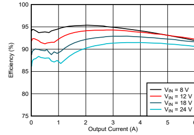
効率 : V OUT = 5V、f sw = 2.1MHz、LM63460-Q1
