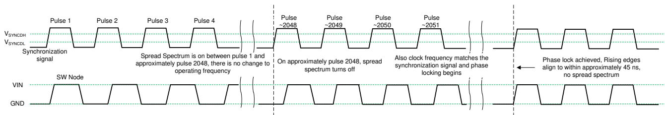
図 7-3. Synchronization Process
