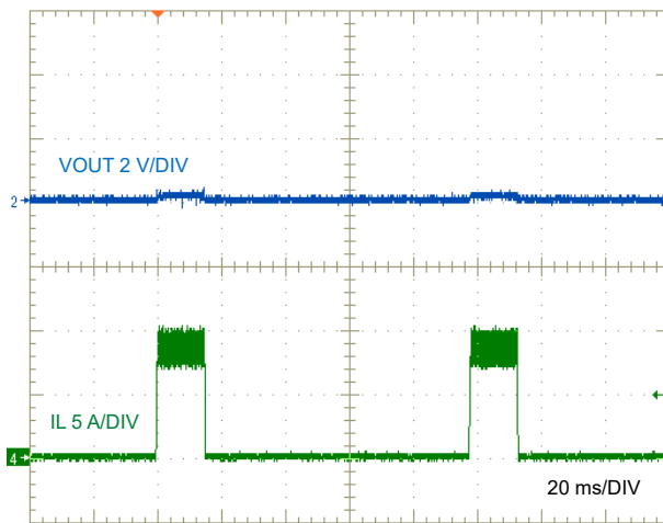
図 8-9. LM634x0-Q1 Short-Circuit Hiccup
