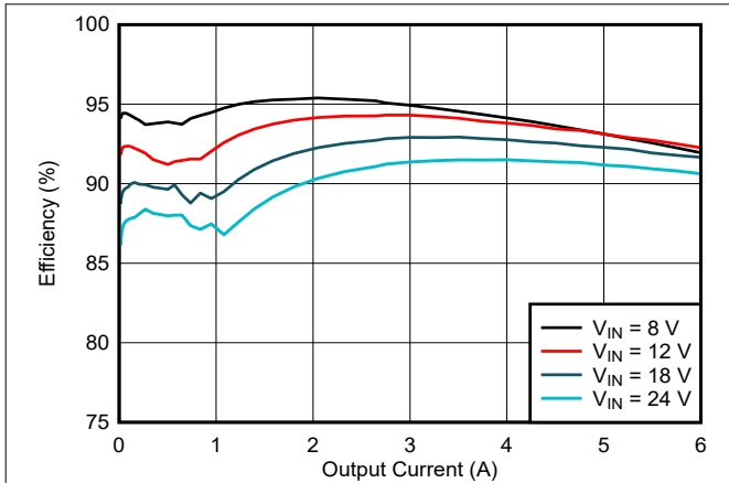
图 8-3. LM644x0-Q1 Efficiency
