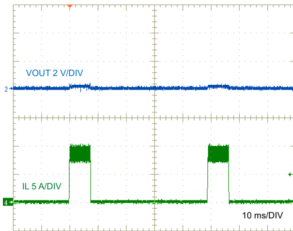
図 8-9. LM644x0-Q1 Short-Circuit Hiccup
