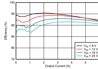
効率 : V_{OUT} = 5V 、 f_{SW} = 2.1MHz 、LM64460-Q1
