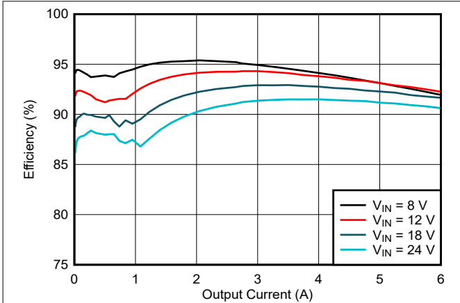
图 8-3. LM644x0-Q1 Efficiency
