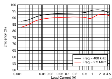
効率と出力電流との関係 ( V_{\text{OUT}} = 5\text{V} , V_{\text{IN}} = 12\text{V} , 自動モード)
