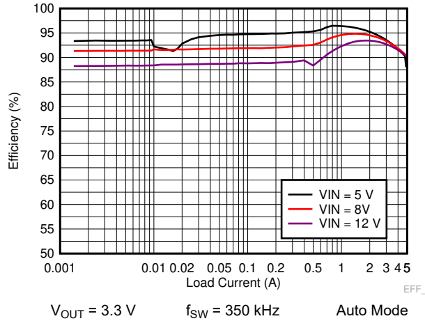
9-9. LM73605-Q1 Efficiency
