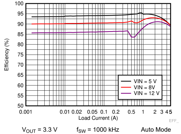
9-10. LM73605-Q1 Efficiency
