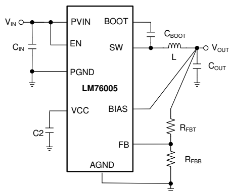
概略回路図
