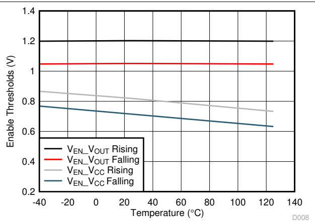
6-4. Enable Threshold
