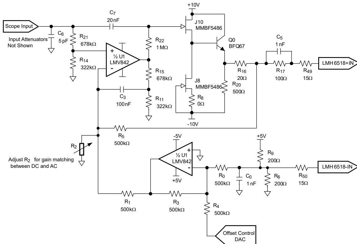
7-11. JFET LNA Implementation
