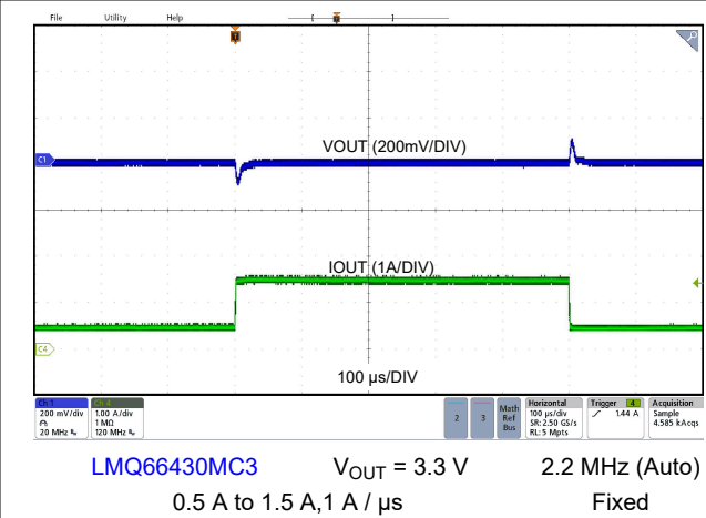
8-11. Load Transient
