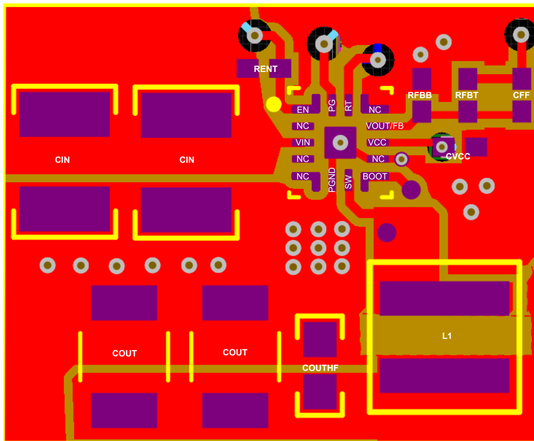
図 8-34. Example Layout
