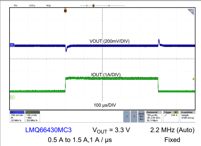
8-11. Load Transient
