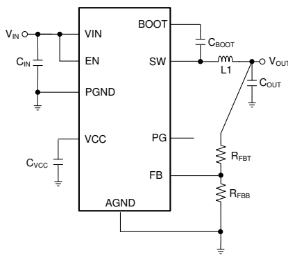
概略回路図
