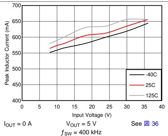
图 6. I PEAK-MIN
