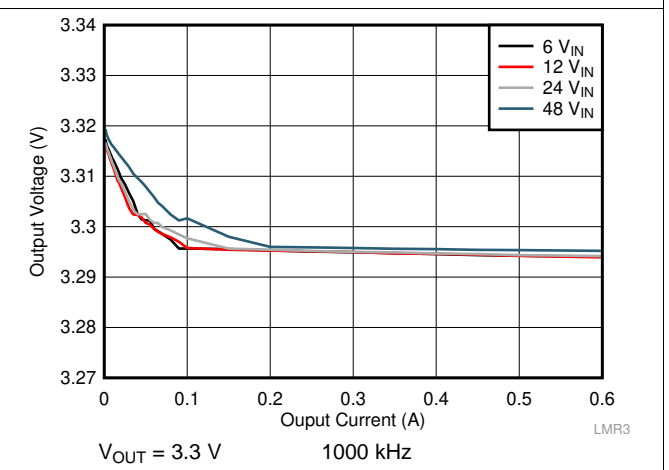
图 24. Load Regulation
