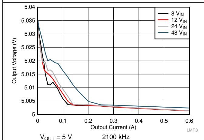
图 45. Load Regulation
