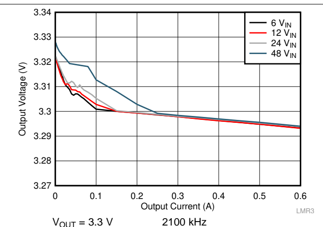
图 46. Load Regulation
