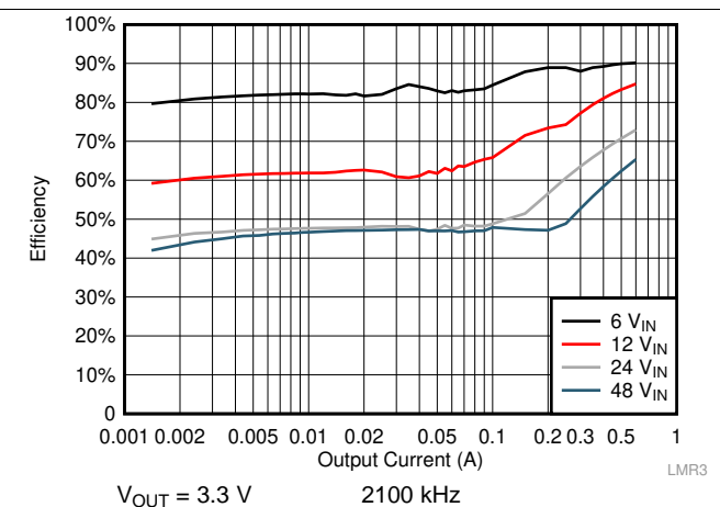
图 44. Efficiency
