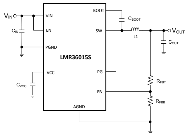
概略回路図
