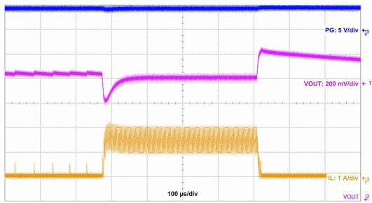
10-16. Load Transient
