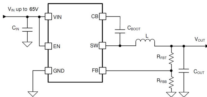
概略回路図
