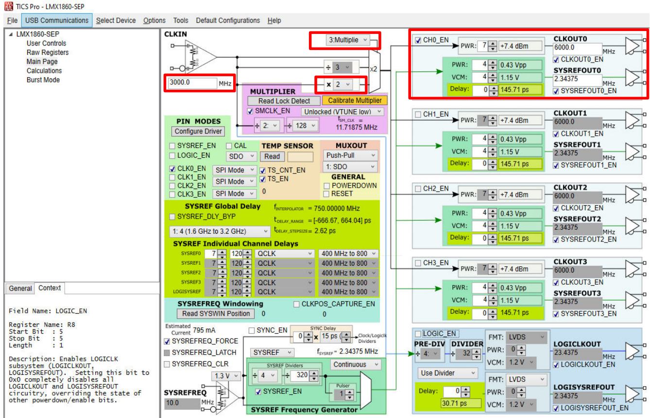
図 7-8. LMX1860-SEP TICS Pro Setup
