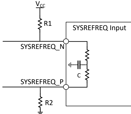
図 6-6. SYSREFREQ Pin Logic Low Setup
