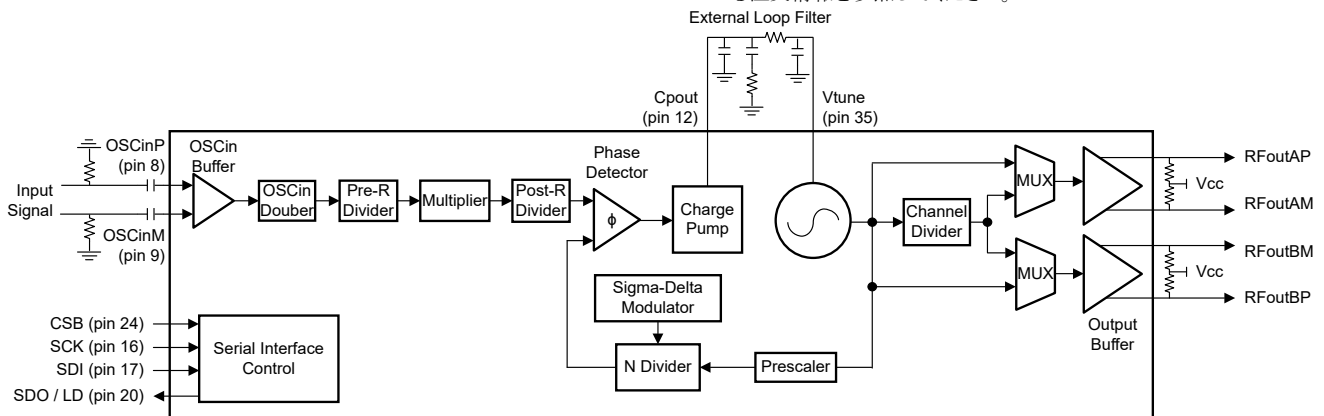
概略回路図
