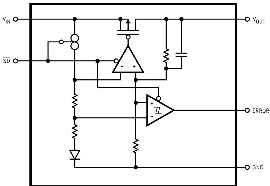
ブロック図 LP3876
