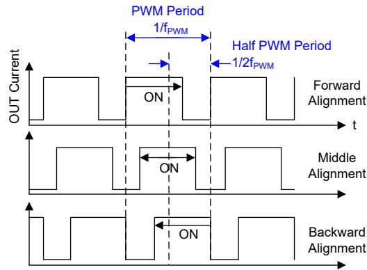
図 8-13. PWM アライメント方式
