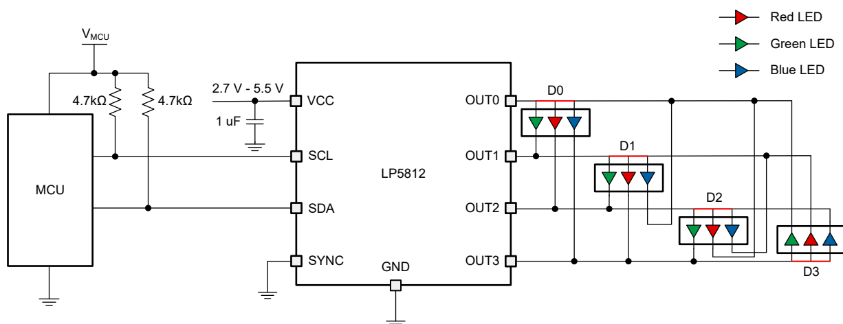
図 7-1. 代表的なアプリケーション - RGB LED を駆動する LP5812
