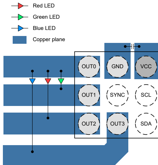
図 9-9. LP5812 DSBGA パッケージのレイアウト例
