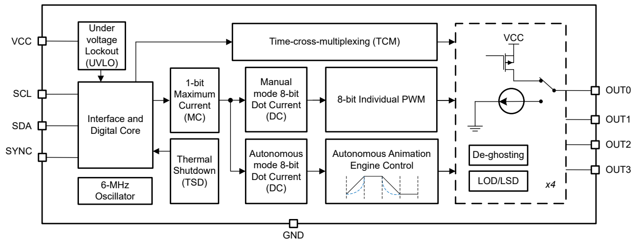
図 8-1. 機能ブロック図
