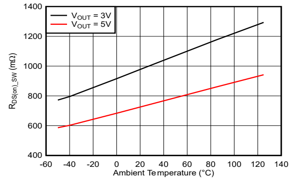
図 5-6. スキャンラインスイッチ MOSFET R_{DS(on)}
