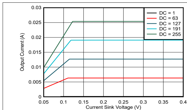
図 5-1. 電流シンク電圧と電流との関係 (MC = 0)
