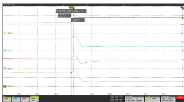
図 7-5. OUT0、OUT1、OUT2、OUT3 のスキャンラインのスイッチング波形
