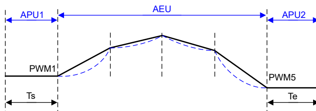
図 6-19. APU の例
