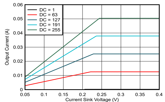
図 5-2. 電流シンク電圧と電流との関係 (MC = 1)
