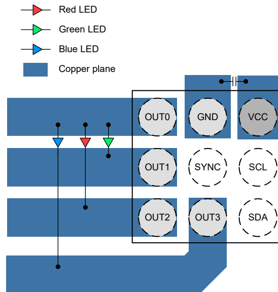
図 7-9. LP5812 DSBGA パッケージのレイアウト例
