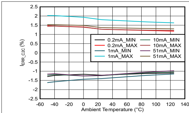
図 5-5. チャンネル間の電流精度と温度との関係 (MC = 1)
