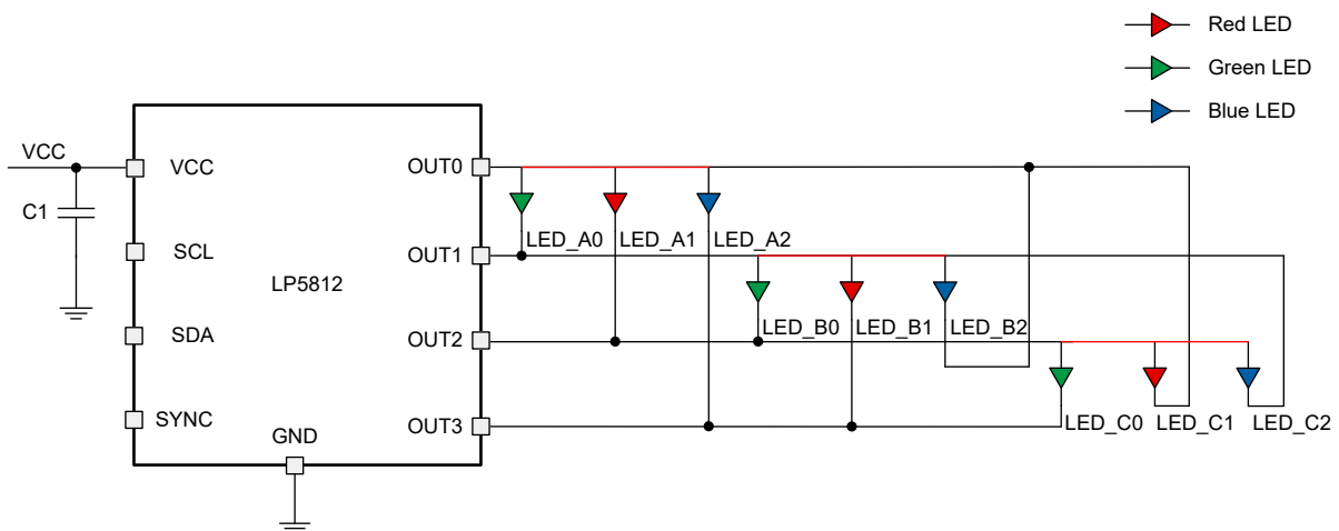
図 8-6. TCM ドライブ・モード、3 スキャン (led_mode = 3h、scan_order_0 = 0h、scan_order_1 = 1h、scan_order_2 = 2h)
