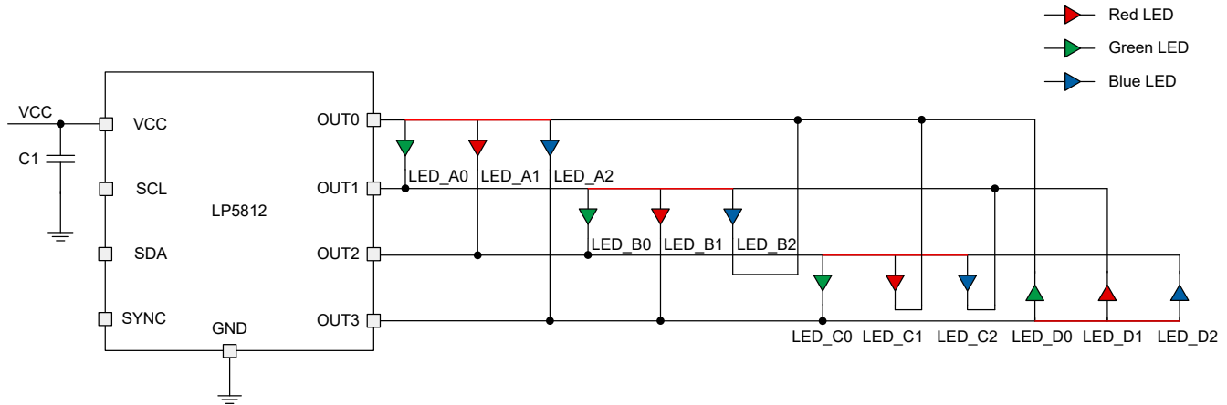
図 6-7. TCM ドライブ・モード、4 スキャン ( \text{led\_mode} = 4\text{h} \text{scan\_order}_0 = 0\text{h} 、 \text{scan\_order}_1 = 1\text{h} 、 \text{scan\_order}_2 = 2\text{h} 、 \text{scan\_order}_3 = 3\text{h} )
