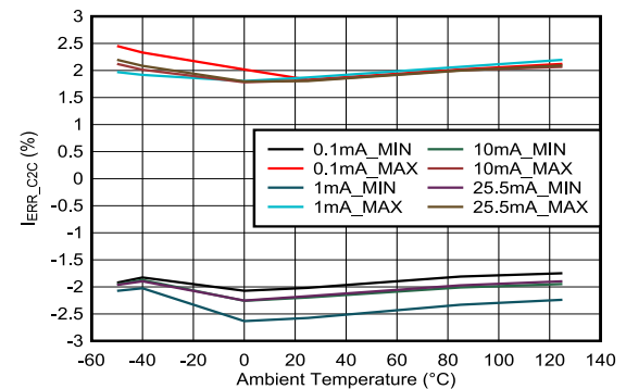
図 5-4. チャネル間の電流精度と温度との関係 (MC = 0)
