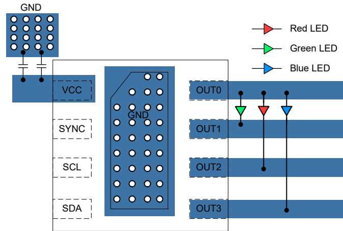
図 9-10. LP5812 WSON パッケージのレイアウト例
