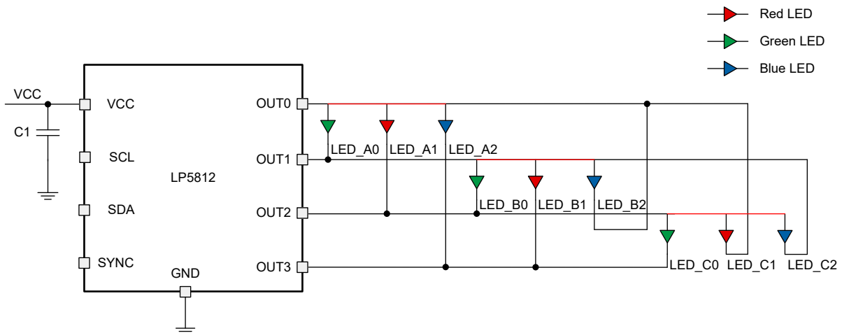
図 6-6. TCM ドライブ・モード、3 スキャン ( led\_mode = 3h 、 scan\_order\_0 = 0h 、 scan\_order\_1 = 1h 、 scan\_order\_2 = 2h )
