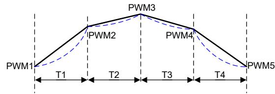
図 8-18. アニメーション エンジン ユニット - 例 2
