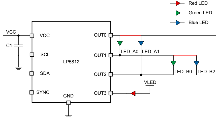
図 8-9. 混在駆動モード、2 スキャン ( led\_mode = 6h , scan\_order\_0 = 0h , scan\_order\_1 = 1h , mix\_sel\_led = 8h )
