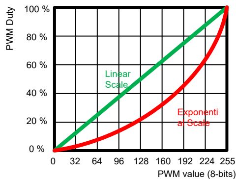
図 8-14. 線形および指数関数 PWM 調光曲線
