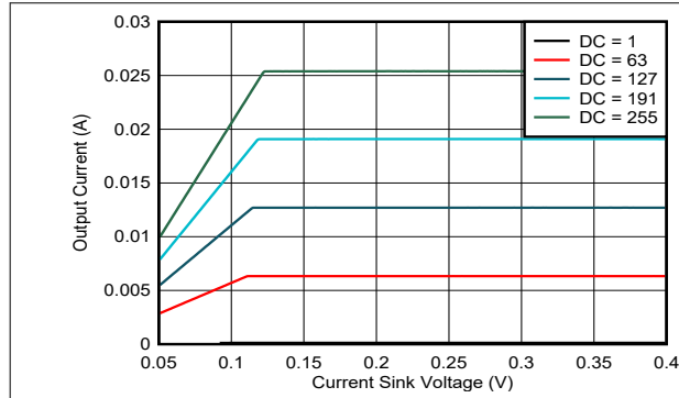
図 7-1. 電流シンク電圧と電流との関係 (MC = 0)
