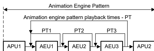
図 6-15. アニメーション エンジン パターン
