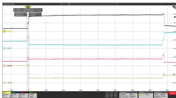
図 7-3. OUT0、OUT1、OUT2、OUT3 のスキャンラインおよび電流シンクの波形
