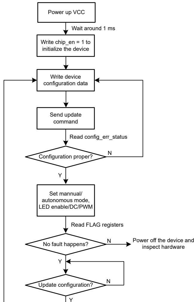
図 7-2. プログラム手順
