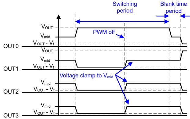
図 8-11. CLAMP_SEL = 1 のときのゴースト除去波形
