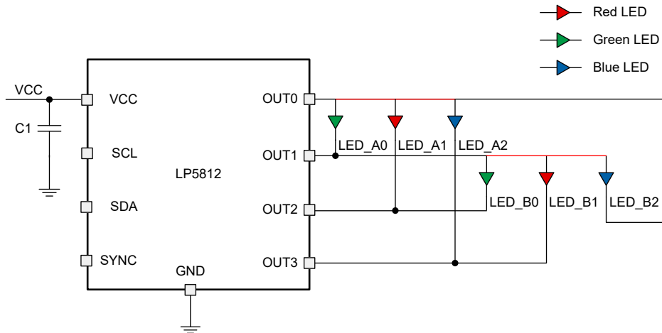
図 8-5. TCM ドライブ・モード、2 スキャン (led_mode = 2h、scan_order_0 = 0h、scan_order_1 = 1h)
