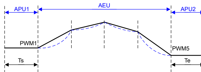
図 8-19. APU の例
