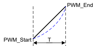
図 8-16. スロープ曲線の例
