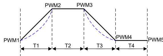
図 6-17. アニメーション エンジン ユニット - 例 1
