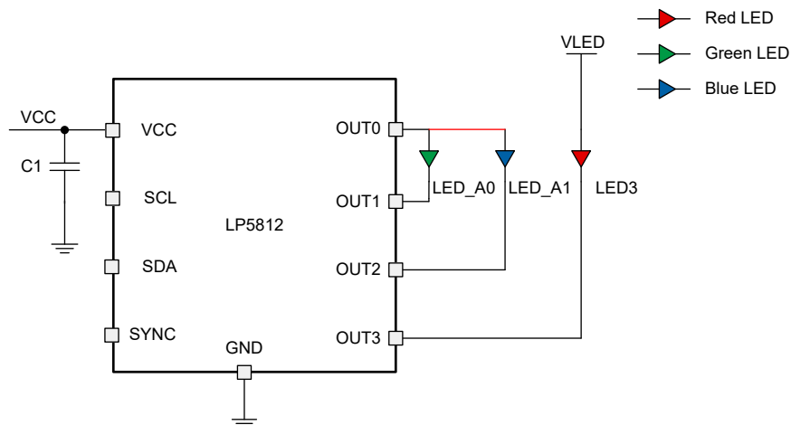
図 6-8. 混在駆動、1 スキャン ( \text{led\_mode} = 5\text{h} 、 \text{scan\_order}_0 = 0\text{h} 、 \text{mix\_sel\_led} = 8\text{h} )
