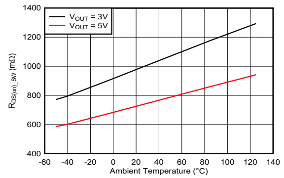
図 7-6. スキャンラインスイッチ MOSFET R_{DS(on)}
