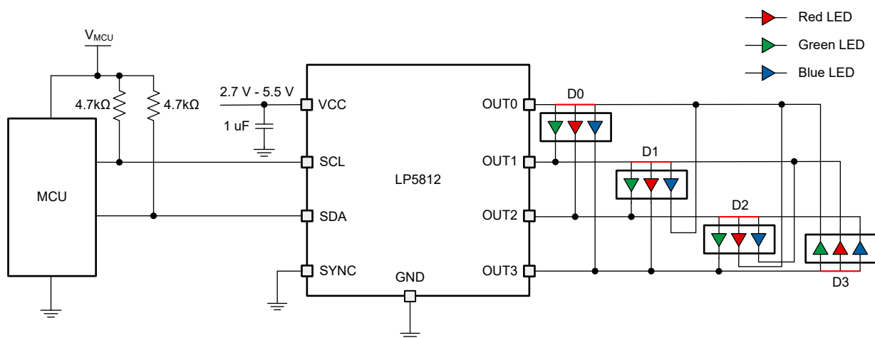
図 9-1. 代表的なアプリケーション - RGB LED を駆動する LP5812
