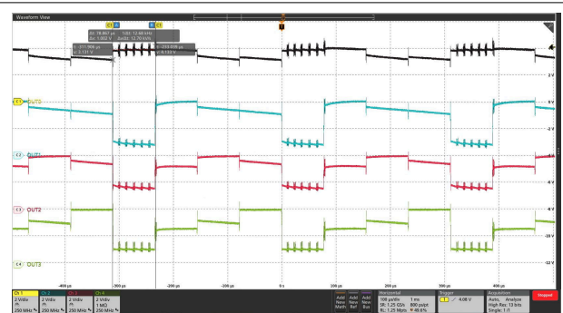
PWM 周波数 = 12kHz LED_A0/A1/A2 イン ーブル led_mode = 4h
