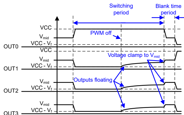
図 6-12. CLAMP_SEL = 0 のときのゴースト除去波形
