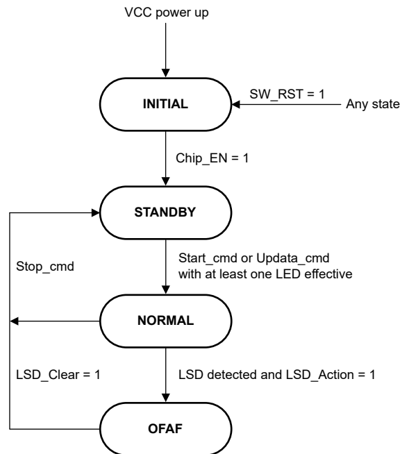
図 6-20. LP5812 の機能モード
