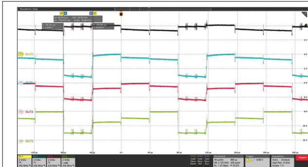
PWM 周波数 = 24kHz LED_A0/A1/A2 イン ーブル led_mode = 4h
