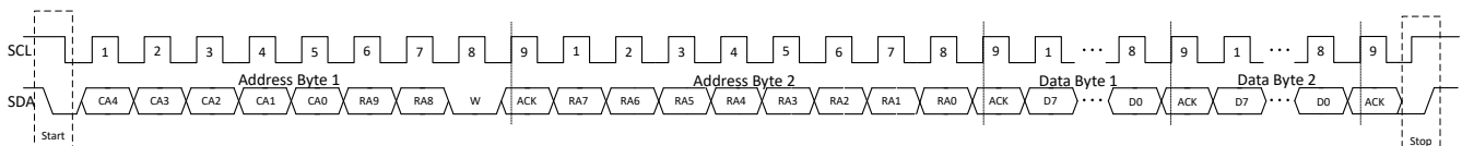
図 6-21. I 2 C 書き込みタイミング
