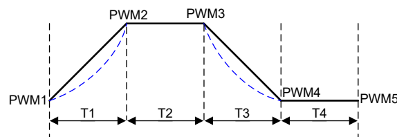
図 8-17. アニメーション エンジン ユニット - 例 1
