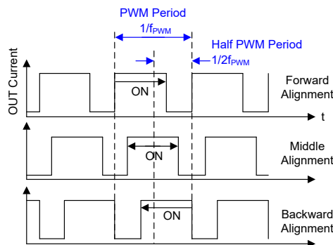
図 6-13. PWM アライメント方式
