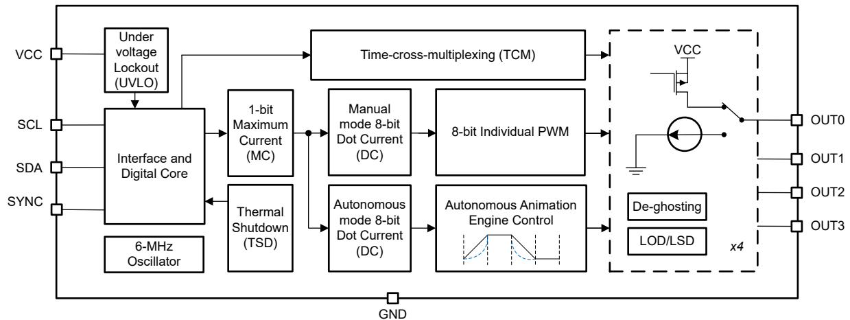
図 6-1. 機能ブロック図
