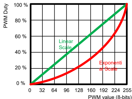
図 6-14. 線形および指数関数 PWM 調光曲線
