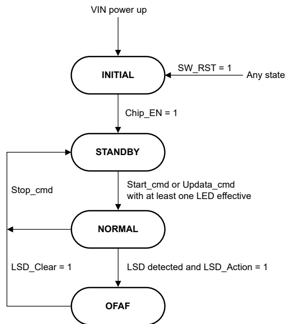
図 8-20. LP5812 の機能モード
