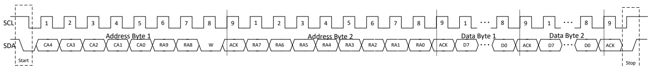
図 8-21. I 2 C 書き込みタイミング
