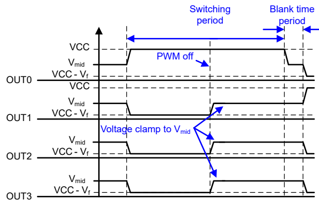
図 6-11. CLAMP_SEL = 1 のときのゴースト除去波形
