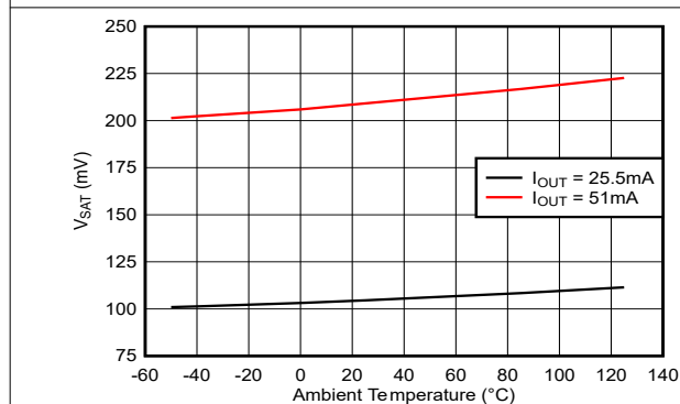
図 5-3. V SAT と温度との関係
