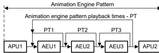
図 8-15. アニメーション エンジン パターン
