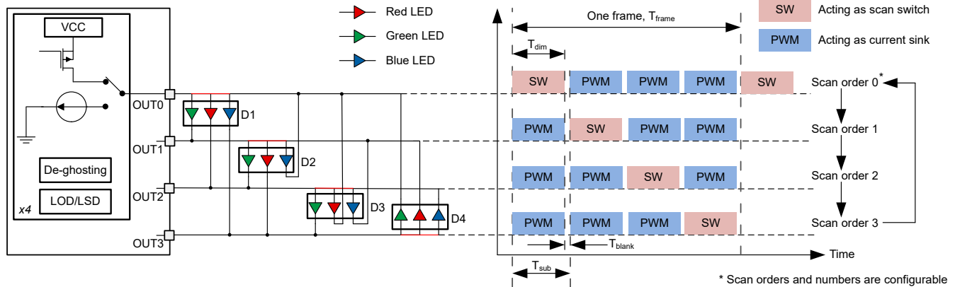
図 8-2 に、4 つの出力の簡略化された TCM 方式のタイミング図を示します。ディスプレイフレーム全体には、4 つのサブ期間が含まれています。各サブ期間には、調光期間とブランク期間が含まれます。スイッチング期間では、1 つの出力がスイッチとして選択され、他の 3 つの出力は電流シンクとして選択されます。ゴーストを除去するため、隣接する 2 つのスイッチング周期の間にブランク時間を適用します。
