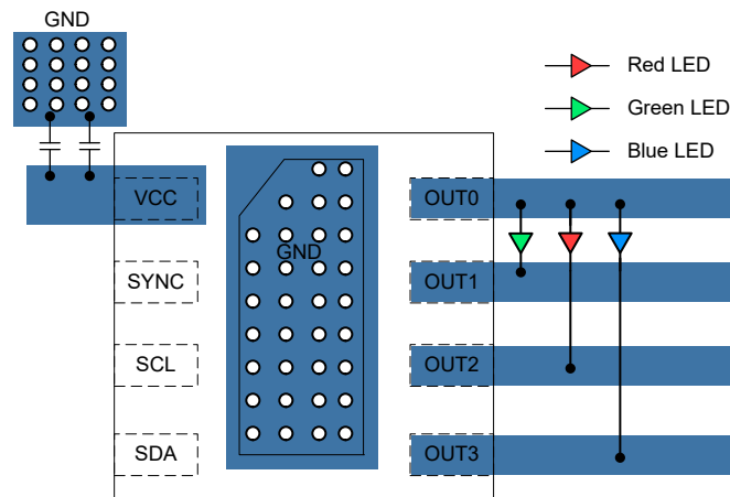
図 7-10. LP5812 WSON パッケージのレイアウト例
