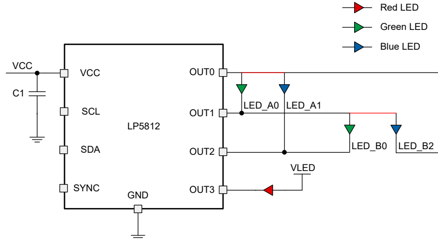
図 6-9. 混在駆動モード、2 スキャン ( led\_mode = 6h , scan\_order\_0 = 0h , scan\_order\_1 = 1h , mix\_sel\_led = 8h )
