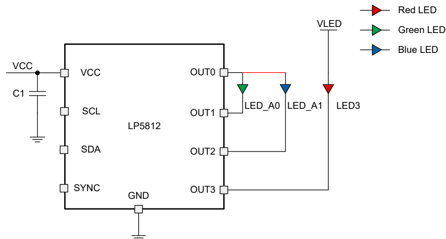
図 8-8. 混在駆動、1 スキャン (led_mode = 5h、scan_order_0 = 0h、mix_sel_led = 8h)
