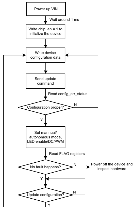
図 9-2. プログラム手順
