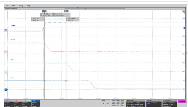
9-5. PWM Phase Shift Enabled
