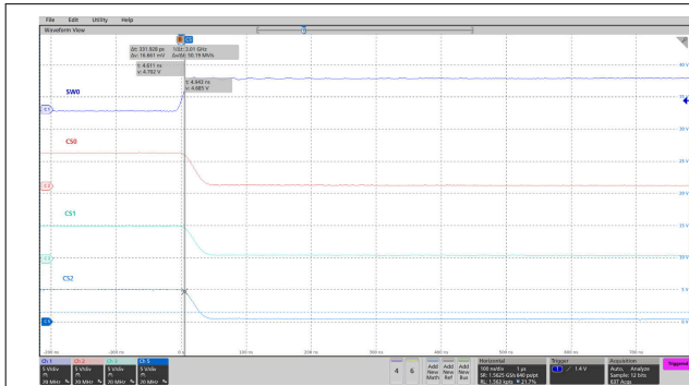
9-4. PWM Phase Shift Disabled
