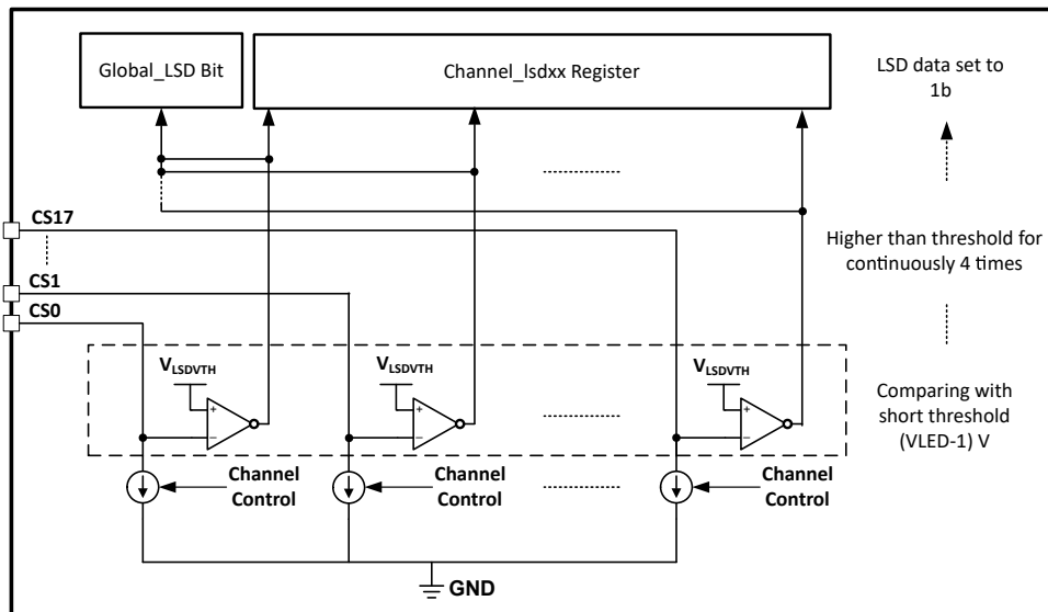
8-9. LSD Circuit
