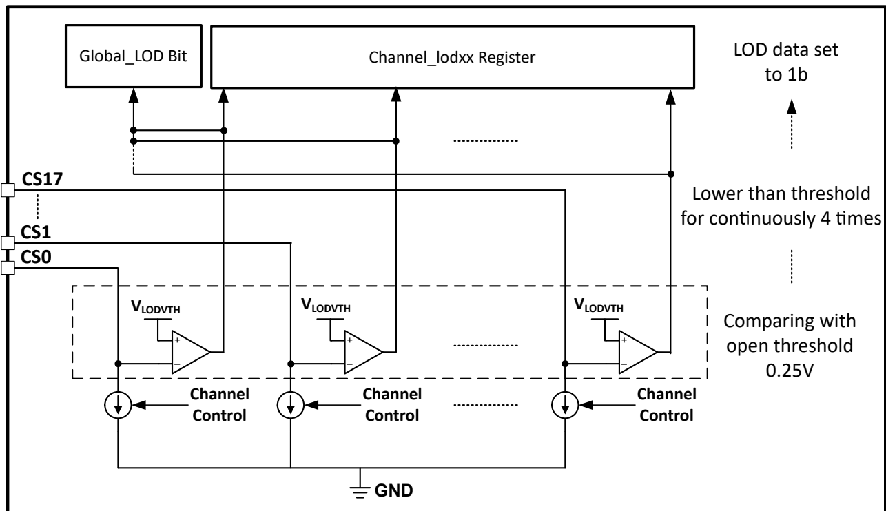
图 7-11. LOD Circuits
