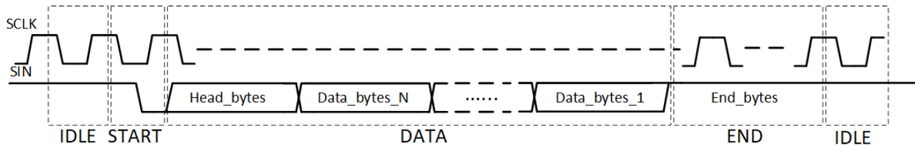
☒ 7-17. CCSI Frame
