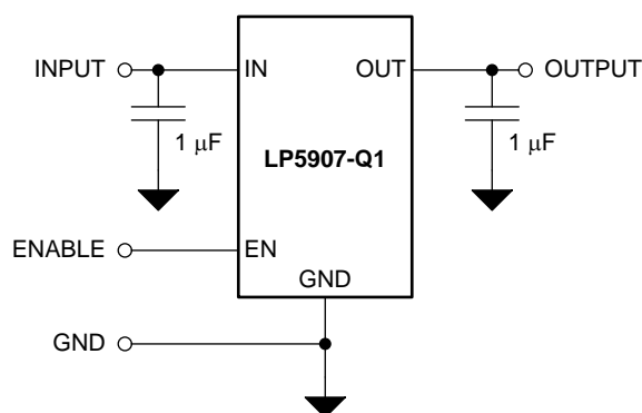
概略回路図
