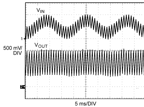
図 7-4. 60Hz Notch Filter Waveform
