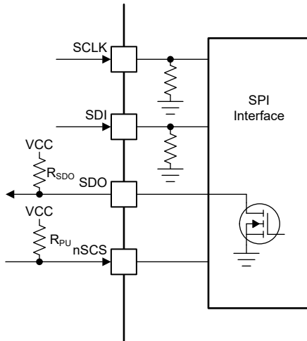
7-7. MCT8314ZZS SPI Interface
