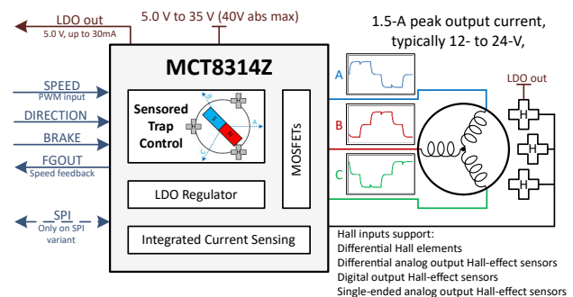
簡略回路図
