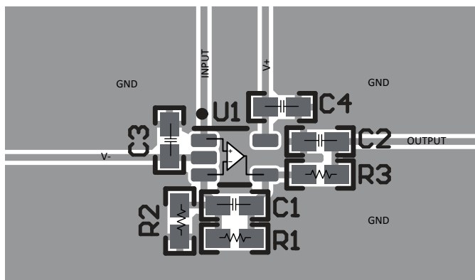
図 8-4. 非反転構成用オペアンプの基板レイアウト - SC70 (DCK) パッケージ
