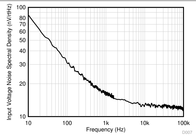
図 6-30. 入力電圧ノイズスペクトル密度
