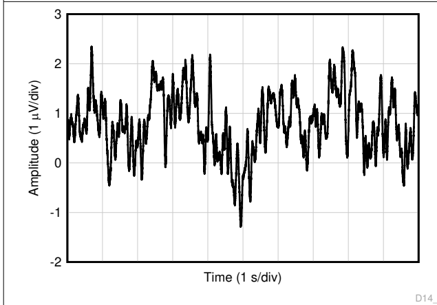
図 6-29. 時間領域での 0.1Hz~10Hz の電圧ノイズ
