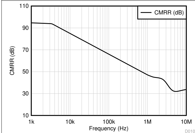
図 6-27. CMRR と周波数との関係
