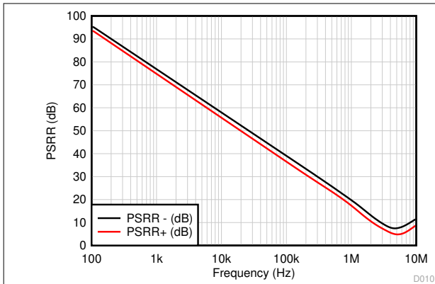
図 6-25. PSRR と周波数との関係
