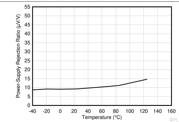
図 6-26. DC PSRR と温度との関係
