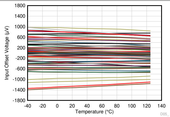
図 6-8. 入力オフセット電圧と温度との関係
