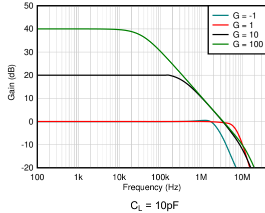
図 6-20. 閉ループゲインと周波数との関係
