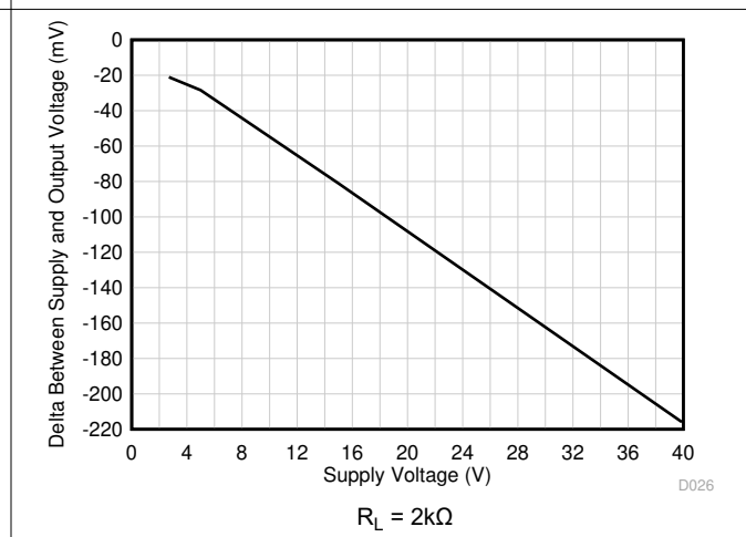
図 6-30. 出力スイングと電源電圧との関係、負のスイング
