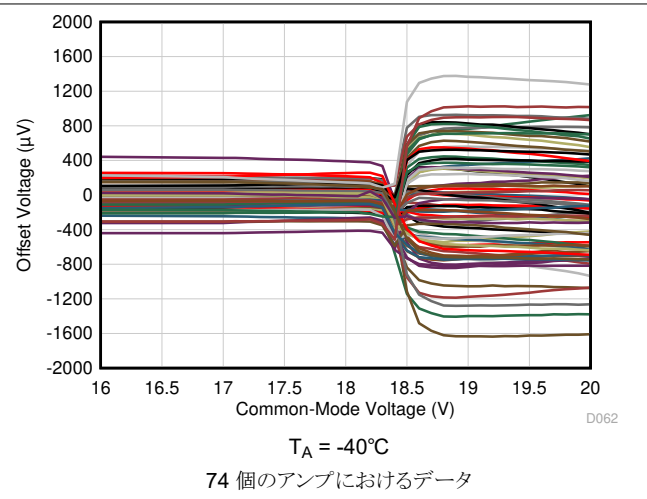
図 5-10. オフセット電圧と同相電圧との関係 (遷移領域)
