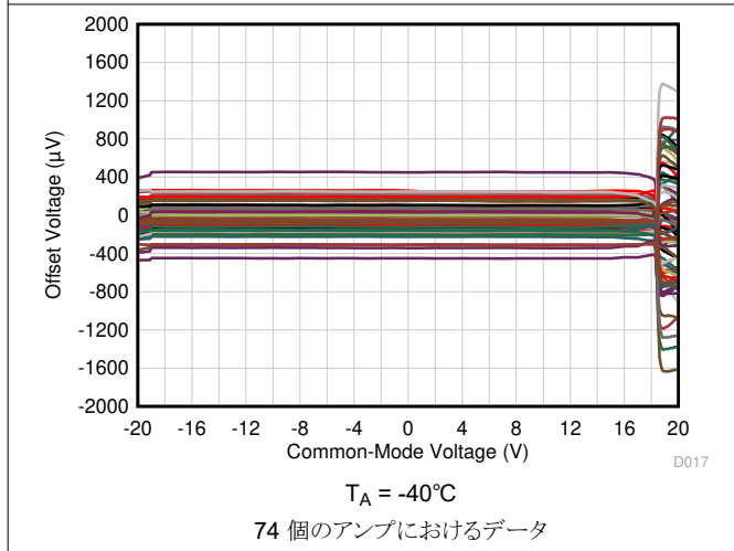
図 5-9. オフセット電圧と同相電圧との関係
