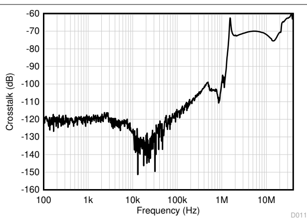
図 5-42. チャンネル セパレーションと周波数との関係
