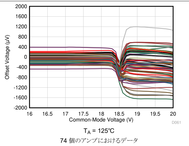
図 5-8. オフセット電圧と同相電圧との関係 (遷移領域)
