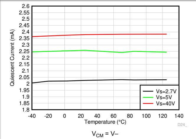
図 5-28. 静止電流と温度との関係
