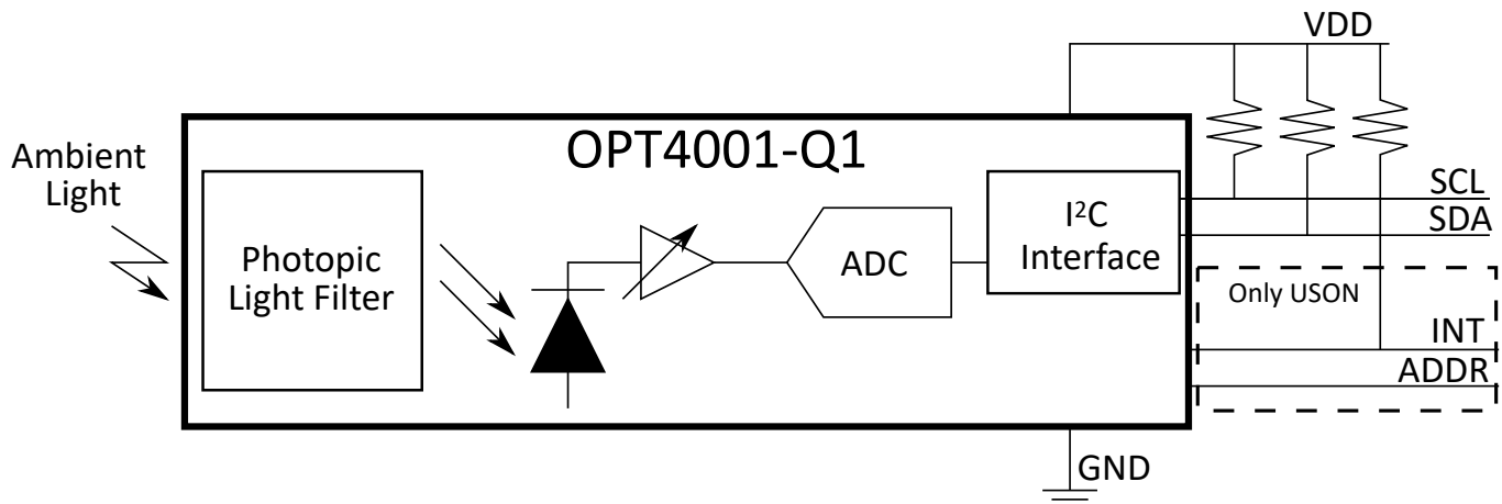
图 6-1. Functional Block Diagram of the OPT4001-Q1
