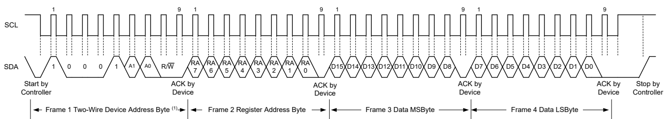
图 6-6. I 2 C Write Example
