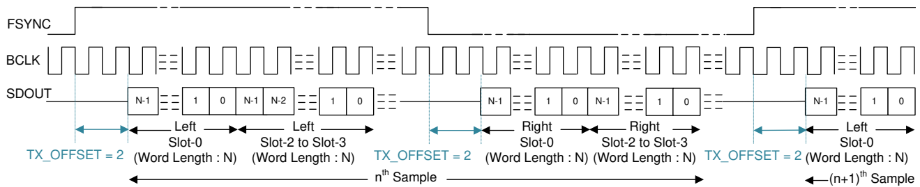
8-11. LJ Protocol Timing (TX_OFFSET = 2)
