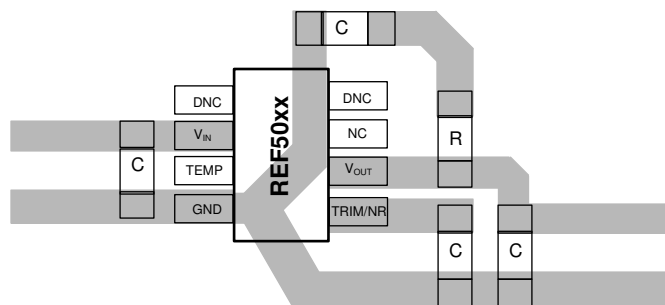
図 12-1. レイアウト例
