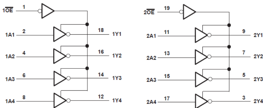
機能ブロック図
