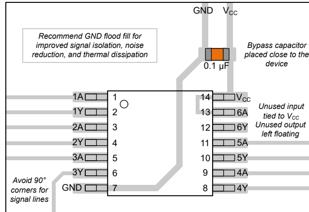
図 8-3. レイアウト例 : SN54SC6T07-SEP
