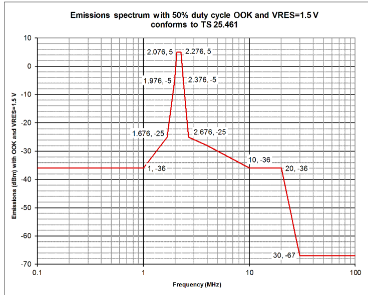
7-3. AISG Emissions Template
