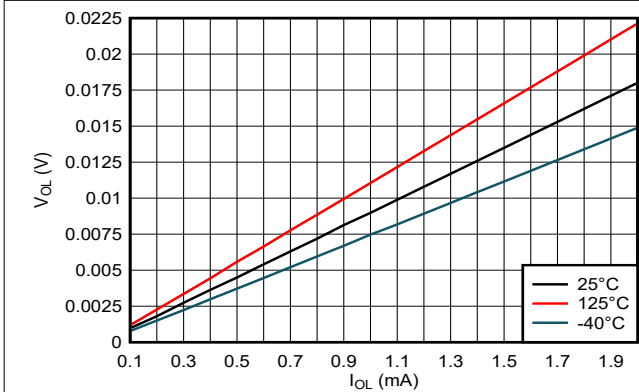
図 5-12. Low 状態における出力電圧と電流との関係、2.5V 電源
