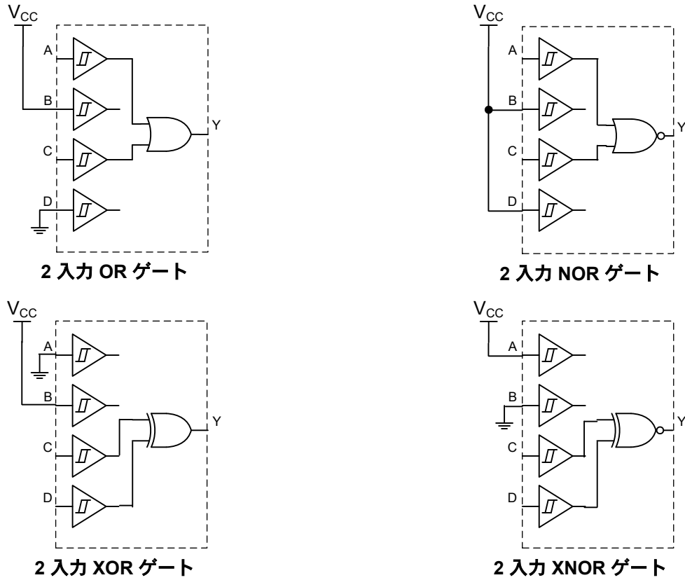
図 7-2. ロジック構成
