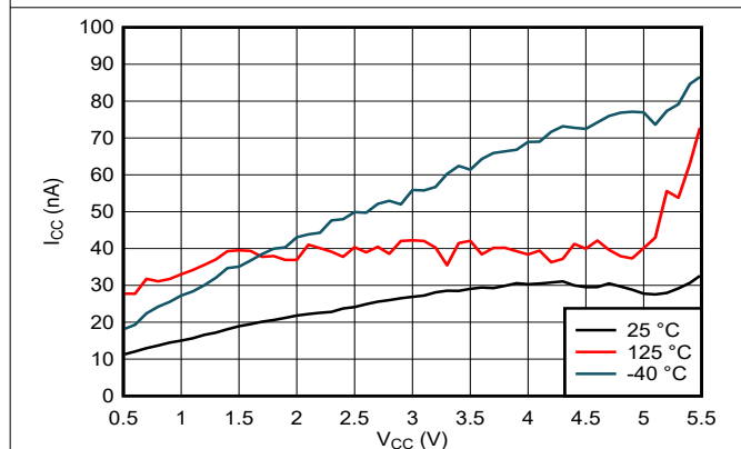
図 5-3. 電源電流と電源電圧との関係
