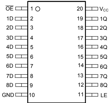
図 4-1. SN74AC573-Q1 PW パッケージ、20 ピン TSSOP (上面図)
