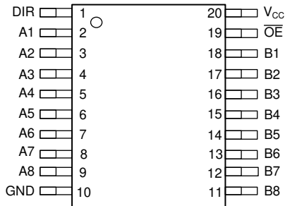
図 4-1. SN74AHC245-Q1 PW パッケージ、20 ピン TSSOP (上面図)
